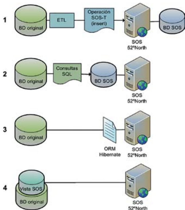
Figura 5. Opciones para el mantenimiento de la base de datos del servicio.
