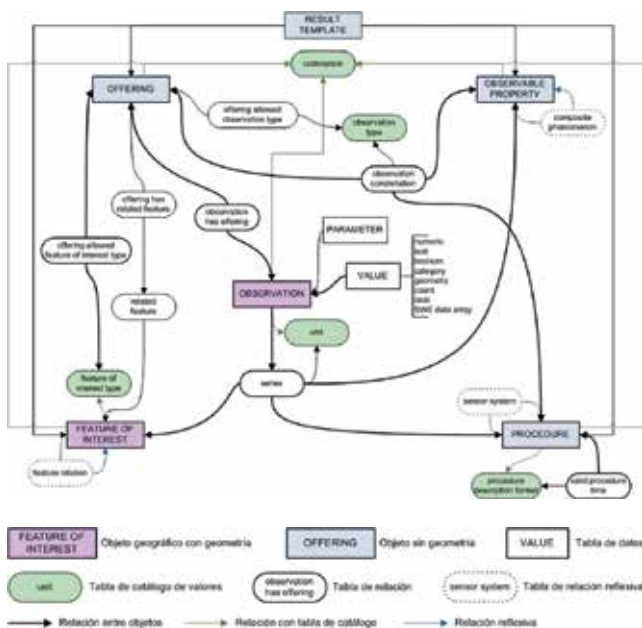
Figura 4. Esquema físico de la base de datos de la aplicación
