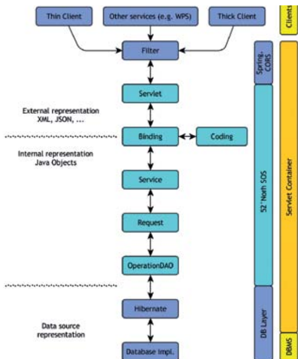
Figura 3. Arquitectura básica de la aplicación
