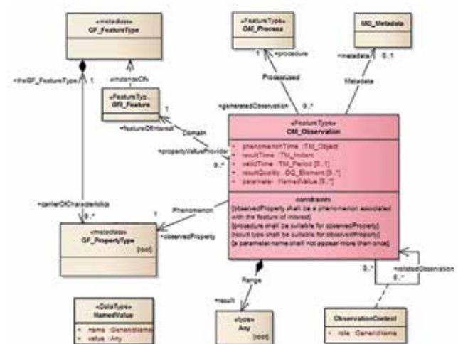
Figura 2. Objeto OM_Observation del esquema de aplicación Observations & Measurements
