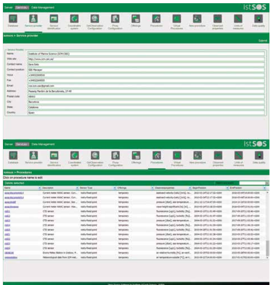
Figura 6. Editor de datos relativos al servicio y a los procedures
