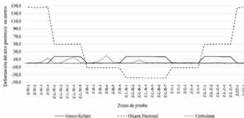
Figura 2. Deformación de un arco geodésico de 50 kilómetros, proyectado a los planos: Gauss-Krüger; Origen Nacional y Cartesiano local
