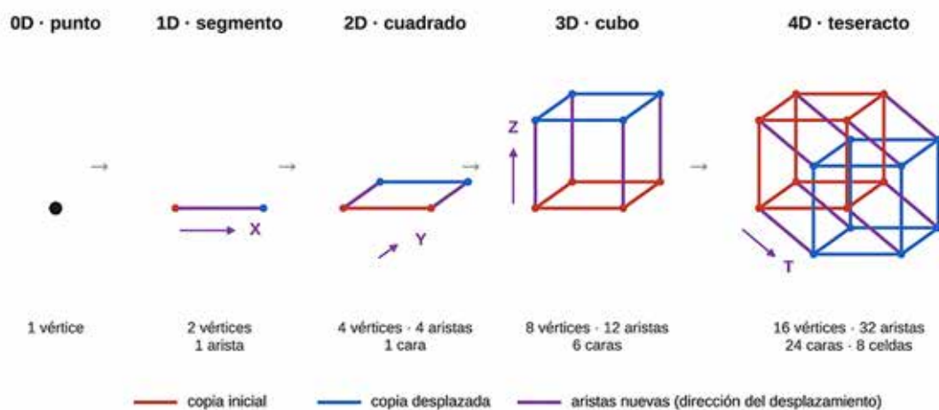
Figura 2. Del punto al tesseracto. Cada figura está formada por dos copias de la anterior (rojo y azul) unidas por aristas en una dirección nueva (morado). El tesseracto son dos cubos unidos por 8 aristas en dirección T .
