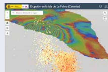
Deformaciones InSAR: fase, entre el 22 de junio y el 20 de septiembre de 2021, en el visualizador 3D de La Palma
