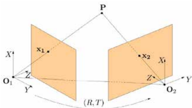
Figura 4. Concepto de paralaje. La visión de un mismo objeto desde dos puntos de vista diferentes permite determinar la profundidad. Fuente: Kleinsteinuber 2014.
